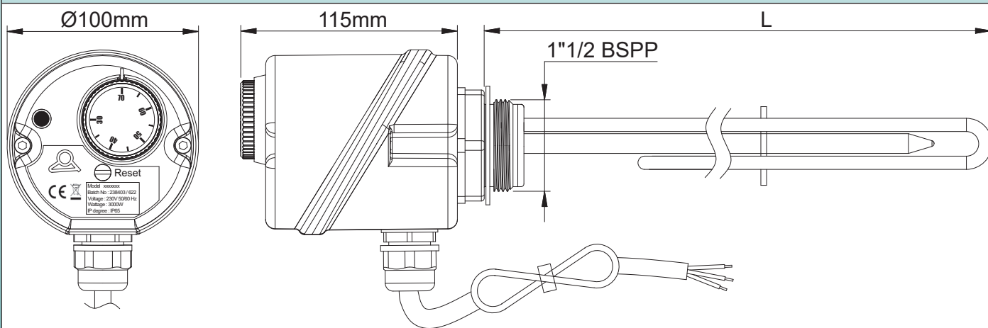
单极 230V 加热器
